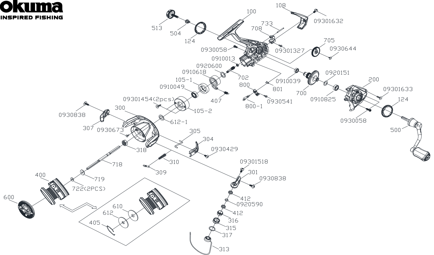
AV-1000B 零件清單
